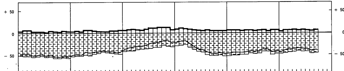
E. — APPRECIATION DU CARNET DE COMMANDES
