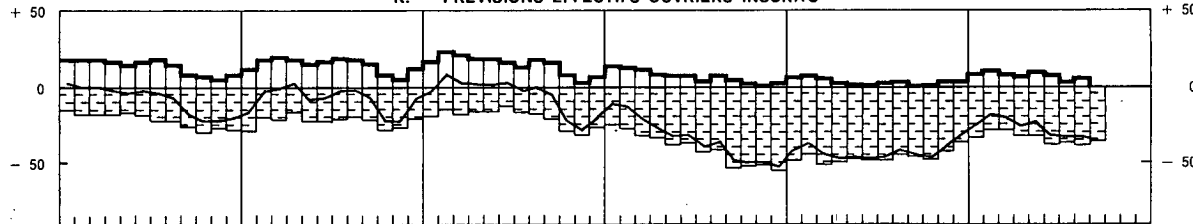
K. — PREVISIONS EFFECTIFS OUVRIERS INSCRITS
